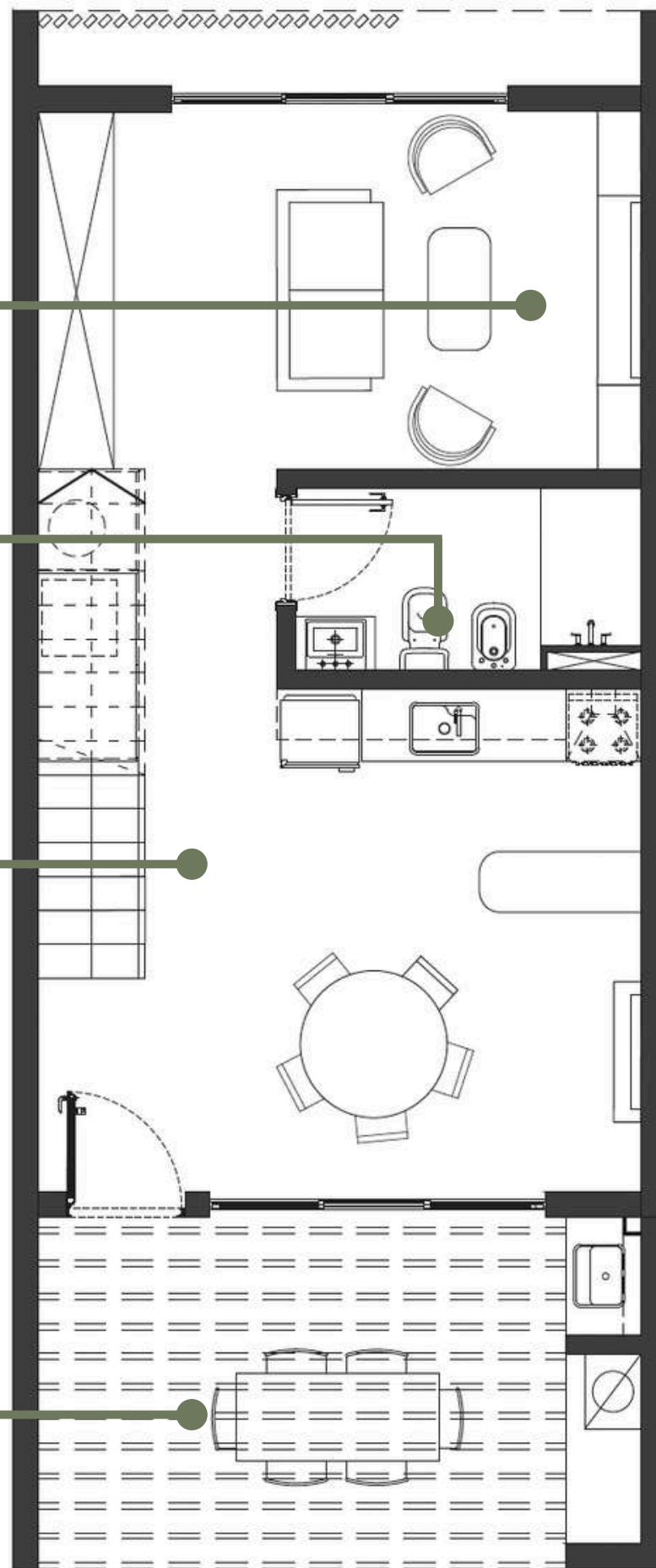
PLANTA BAJA
