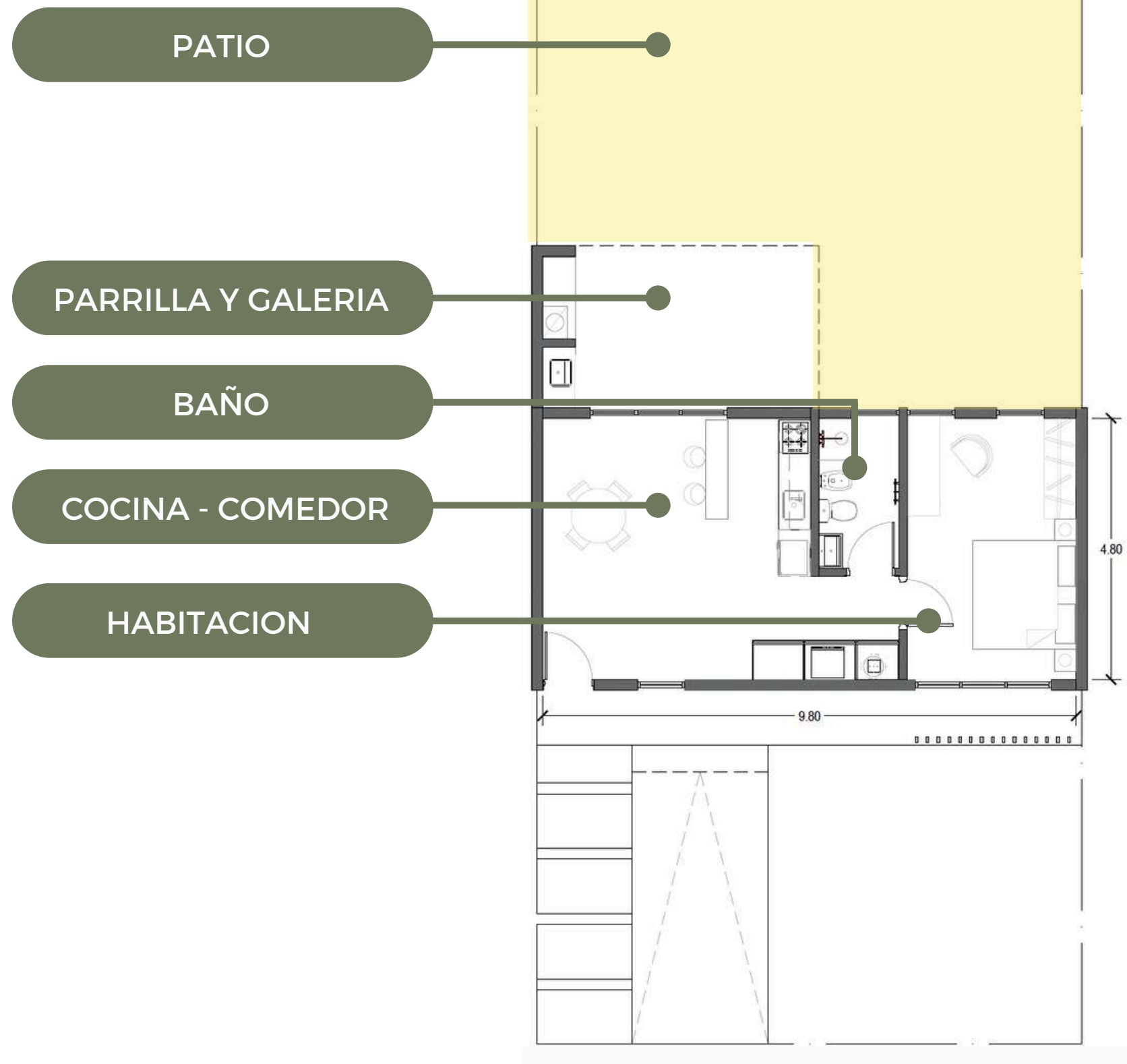
PLANTA BAJA
