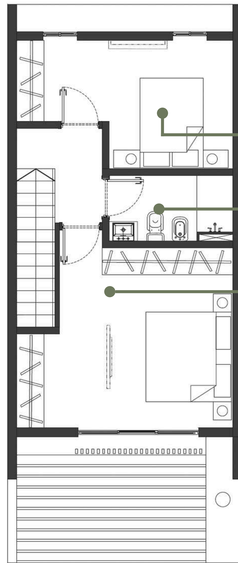
PLANTA ALTA
