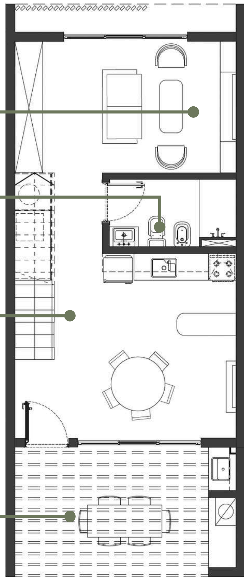
PLANTA BAJA
