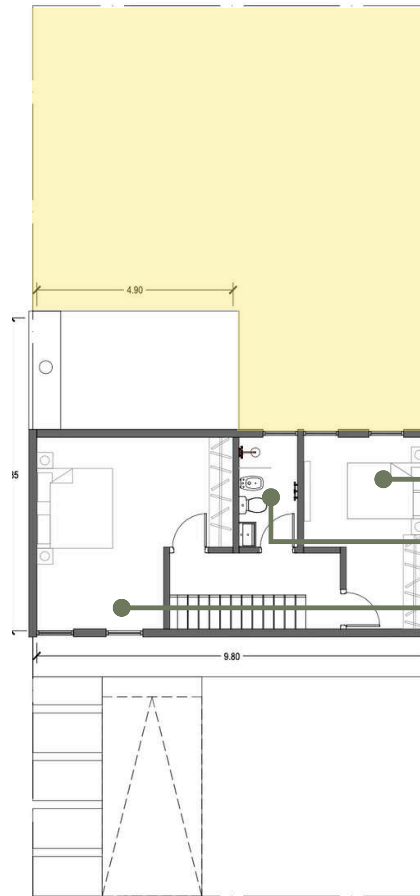
PLANTA ALTA
